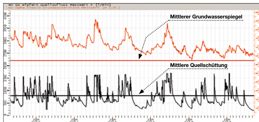
Die Grafik zeigt den Grundwasserstand (rot) sowie die Quellschüttungsmenge der letzten Jahre (schwarz)
